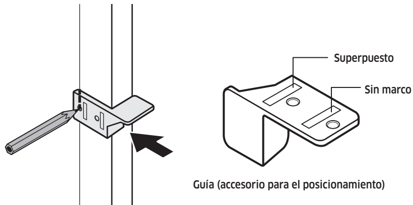
Tipo superpuesto
