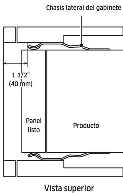
Tipo superpuesto
