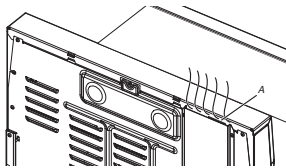
A. Ducto de ventilación del horno
